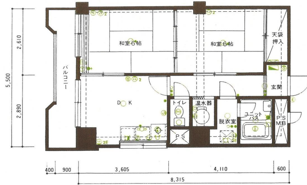
間取図
